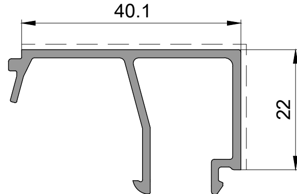
P 1497 Çıta Profili / 0,435kg/mt Glazing Bead Profile
