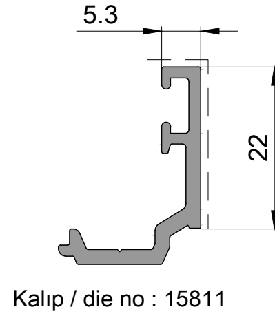
P 1647 Çıta Profili / glazing bead profile 0,275kg/mt
