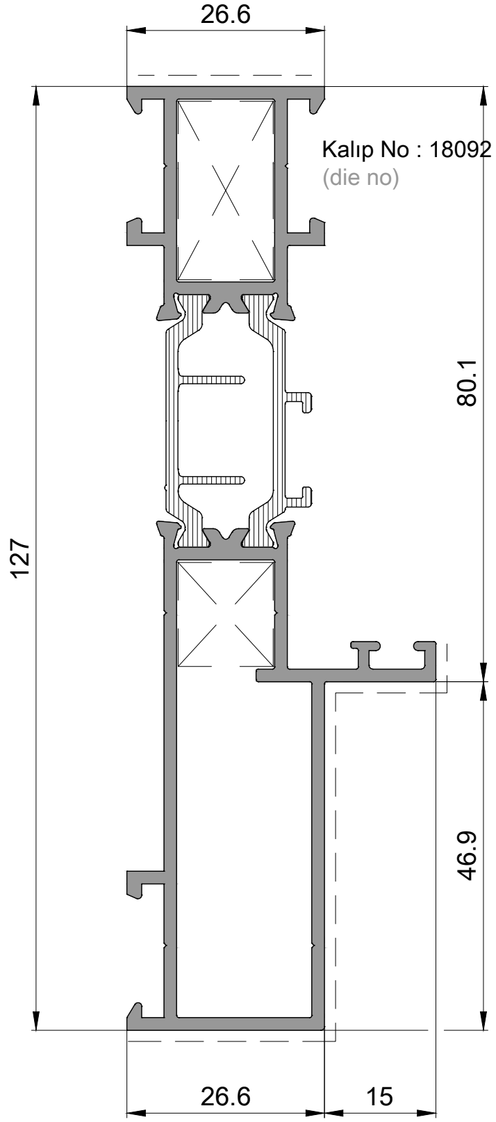
P 2503 Yan Düşey Profil / Side Mullion 1,830kg/mt
