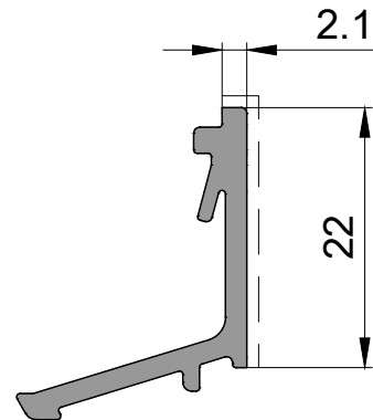
P 1496 Çıta Profili / 0,245kg/mt Glazing Bead Profile
