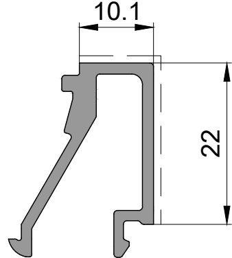
P 1494 Çıta Profili / 0,325kg/mt Glazing Bead Profile
