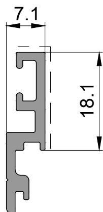
P 2414 Çıta Profili / glazing bead profile 0,235kg/mt
