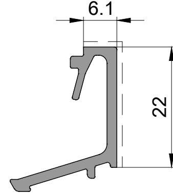
P 1495 Çıta Profili / 0,270kg/mt Glazing Bead Profile
