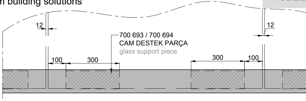
DIŞ GÖRÜNÜŞ EXTERNAL VIEW
