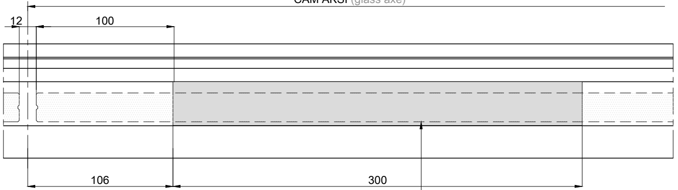
ÜST GÖRÜNÜŞ TOP VIEW
