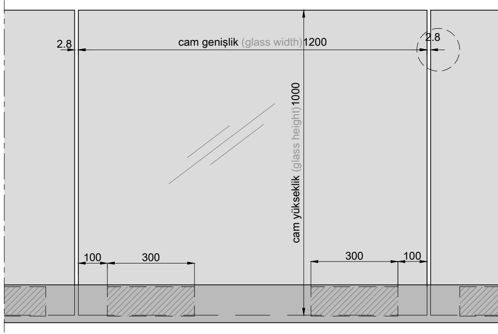
DIŞ GÖRÜNÜŞ EXTERNAL VIEW
