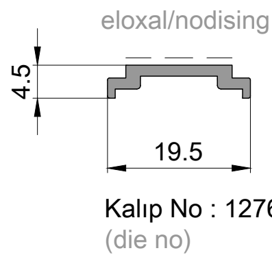
P 1020 Tij Profili / Rod Profile 0,105kg/mt
