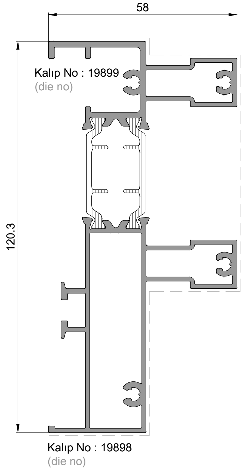
P 2564 Üst Kasa Profili Top Frame Profile 2,160kg/mt
