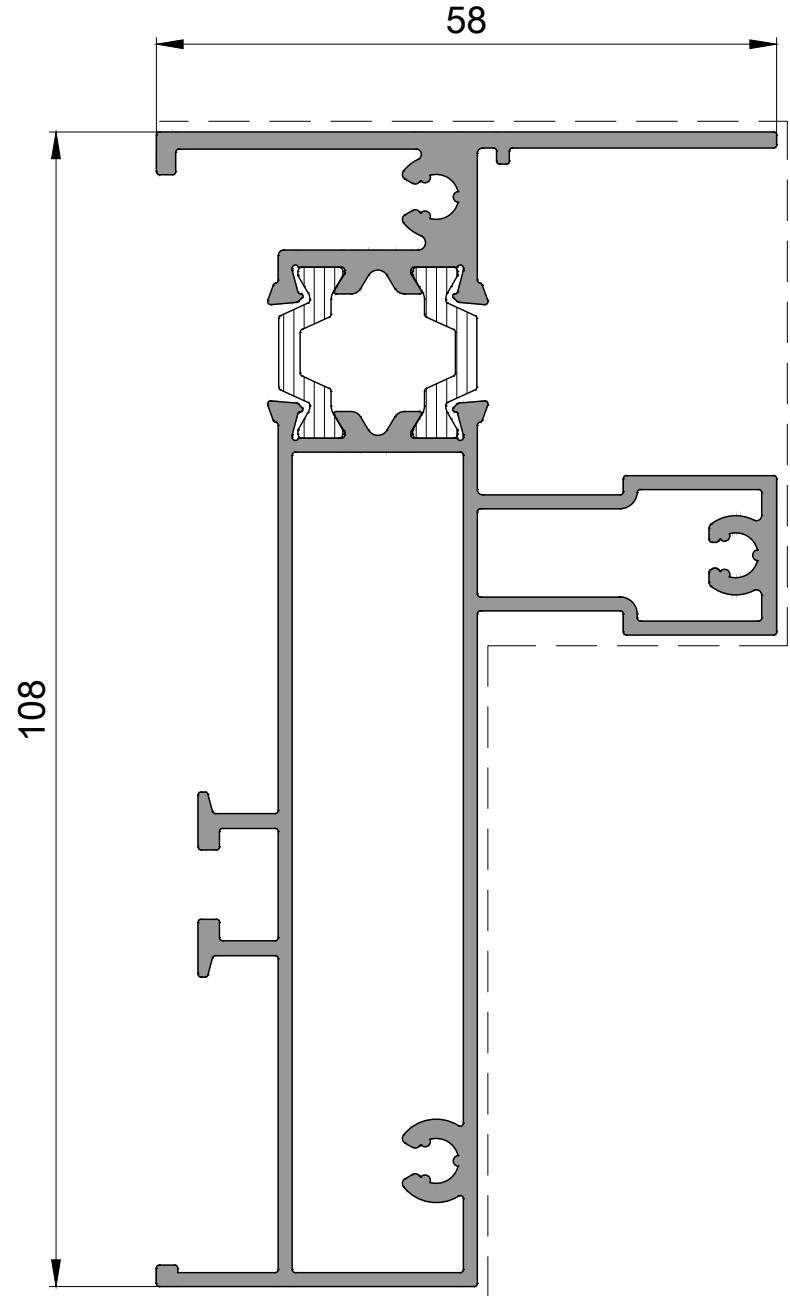
P 2574 Üst Kasa Profili Top Frame Profile 1,910kg/mt
