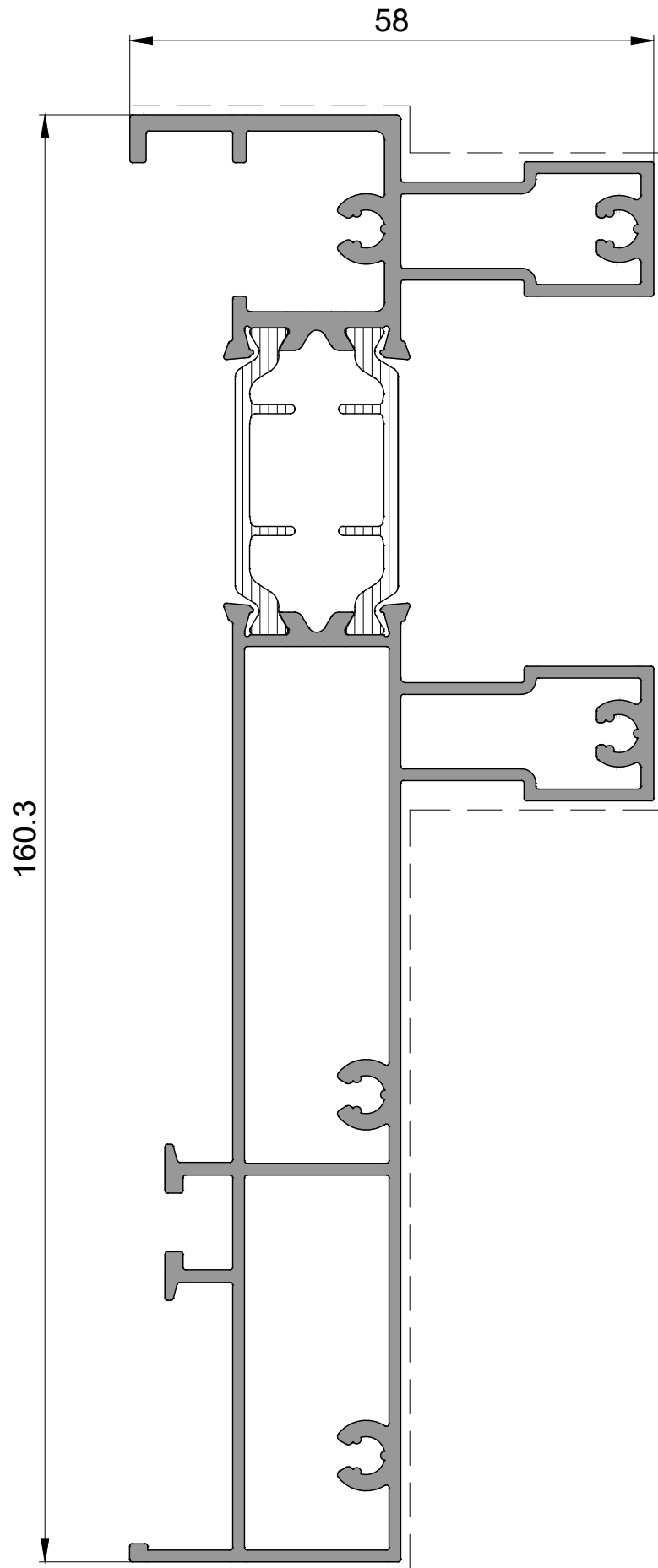
P 2565 Üst Kasa Profili Top Frame Profile 2,560kg/mt
