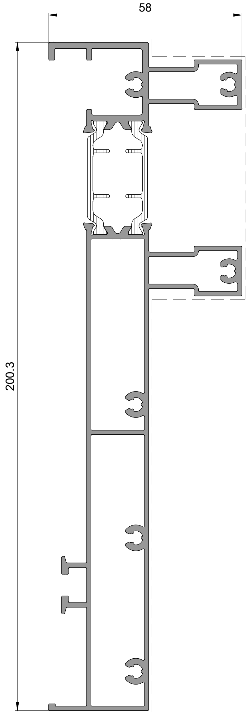
P 2566 Üst Kasa Profili Top Frame Profile 2,910kg/mt
