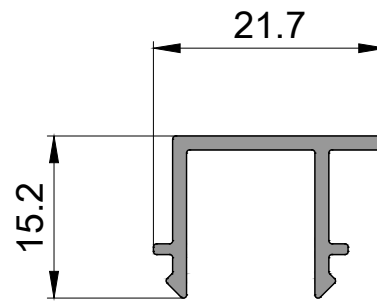
P 2556 Kapak Profili Cap Profile 0,180kg/mt
