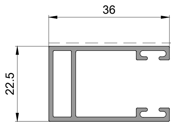
P 2557 Panjur Kanal Profili Roller Rail Profile 0,450kg/mt
