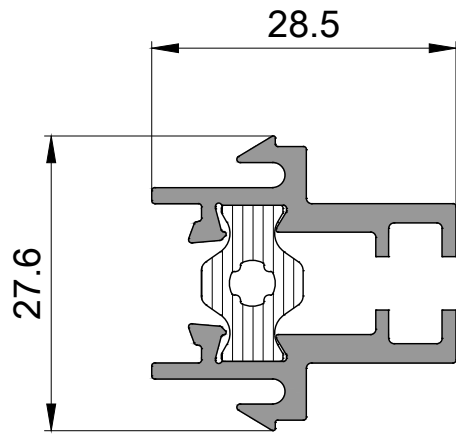
P 2555 Adaptör Profili Adepter Profile 0,600kg/mt
