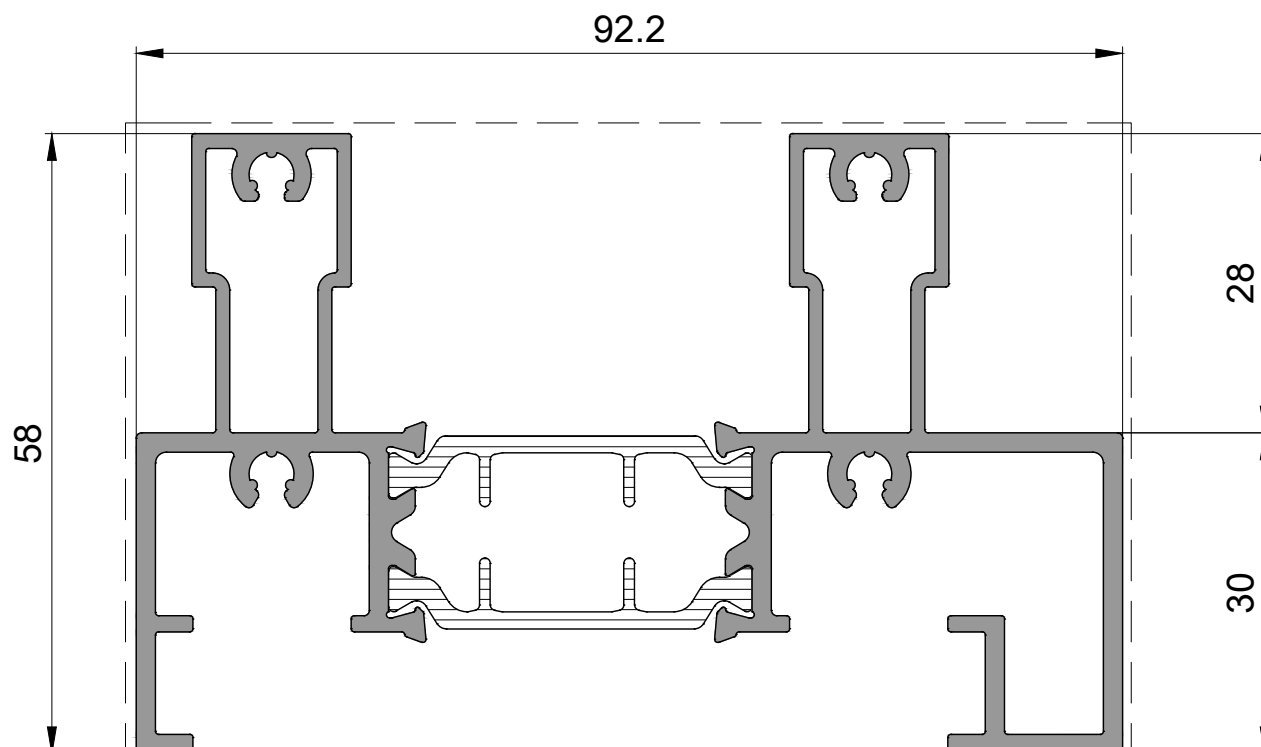
P 2590 Üst Kasa Profili Top Frame Profile 2,000kg/mt
