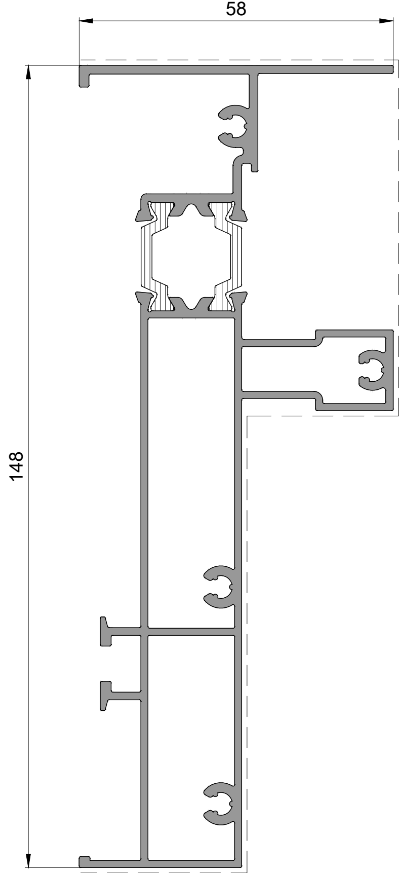
P 2578 Üst Kasa Profili Top Frame Profile 2,275kg/mt
