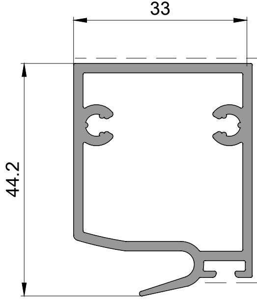
P 2577 Dış Kenet Profili External Interlock Profile 0,860kg/mt
