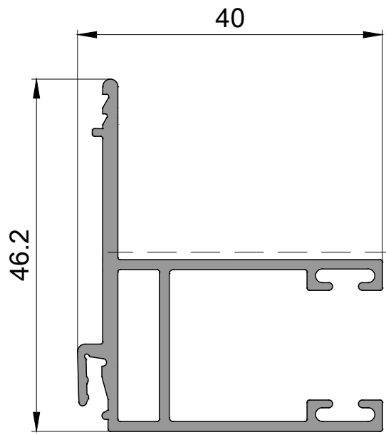
P 2591 Panjur Kanal Profili Roller Rail Profile 0,645kg/mt
