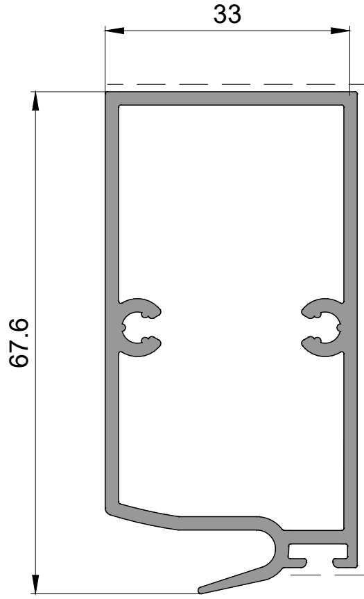
P 2581 Dış Kenet Profili External Interlock Profile 1,090kg/mt
