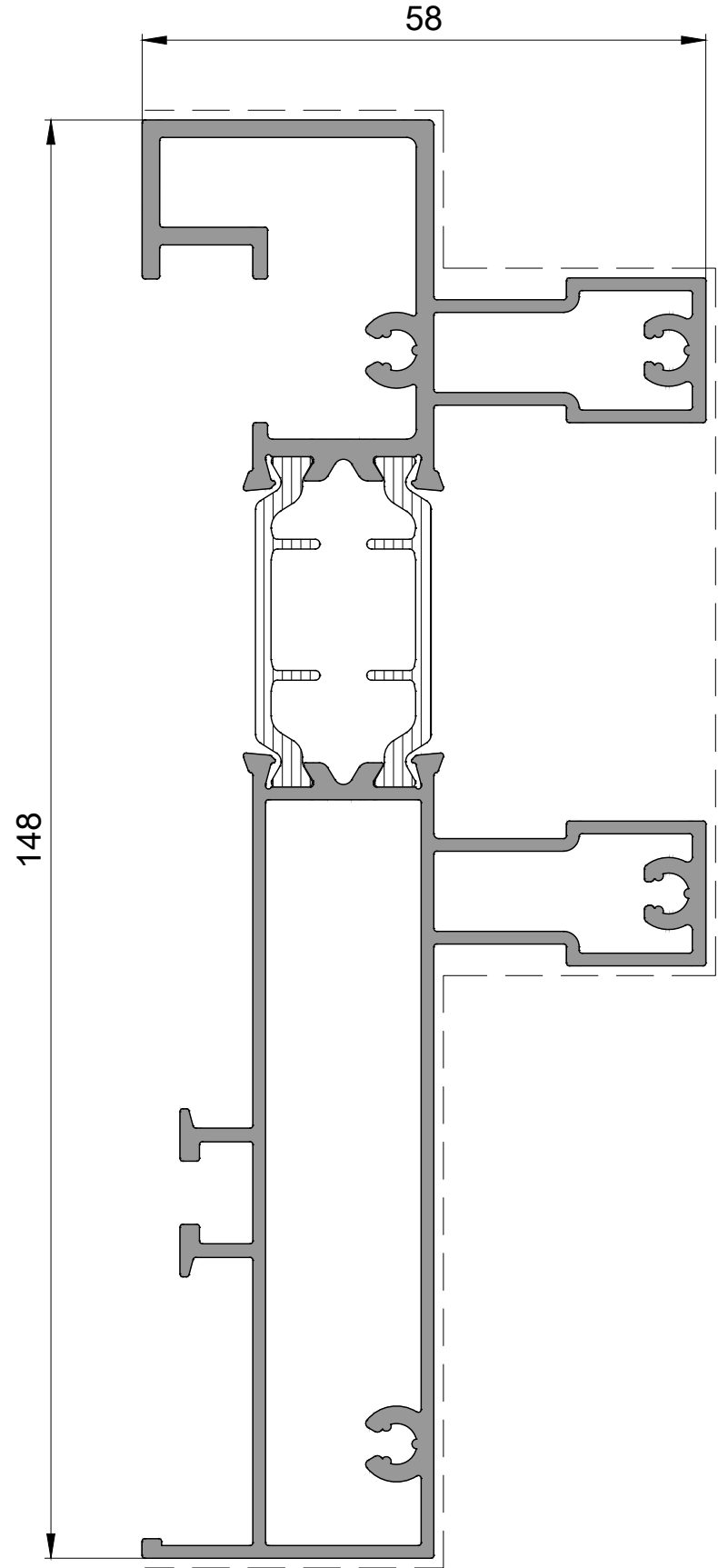
P 2582 Üst Kasa Profili Top Frame Profile 2,440kg/mt
