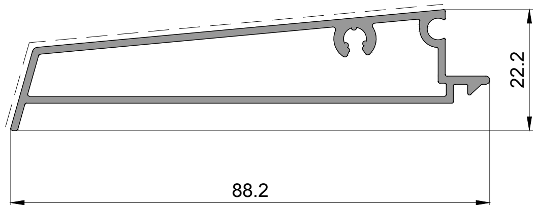
P 2636 Denizlik Profili / Piece D'appui 0,765kg/mt
