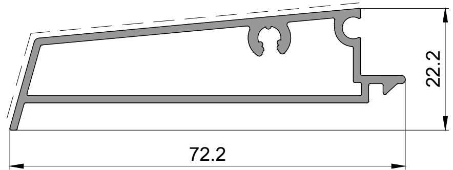
P 2635 Denizlik Profili / Piece D'appui 0,660kg/mt
