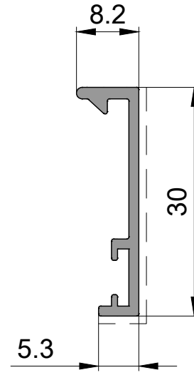
P 2633 Pervaz Profili / Aile De Recouvrement 0,170kg/mt
